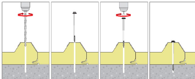
Montagens em betão
