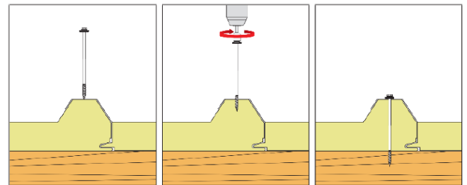
Montagens em madeira
